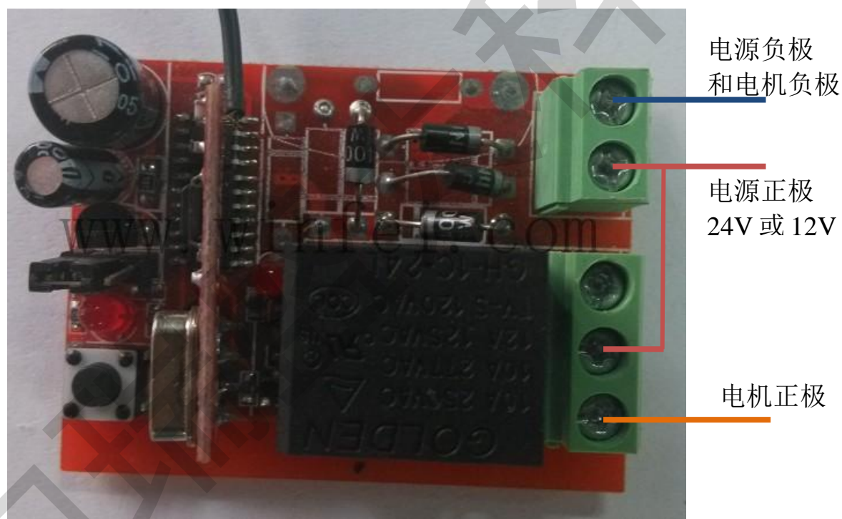
交流&直流电机点动/锁存控制接法（图 1）
